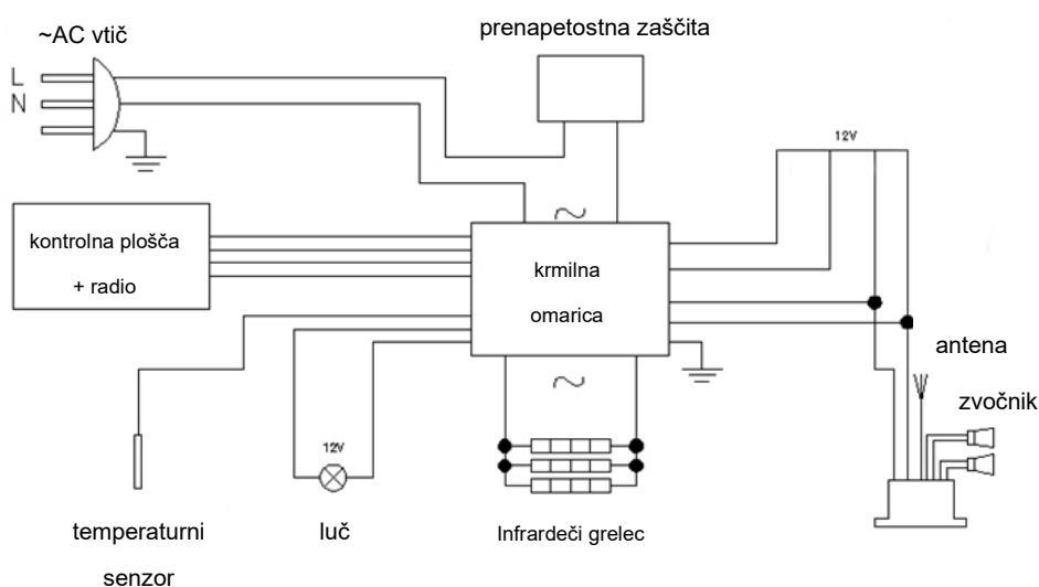
shema tokokroga
